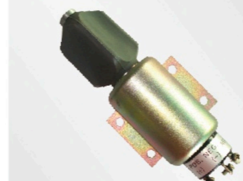
YK025 12V/24V OE:2003-24E7U1B1S2A 适用:康明斯/工程机械 For:Cummins
