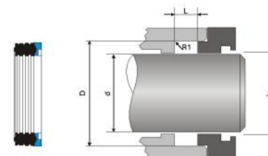
规格及沟槽尺寸 specification & groove size
