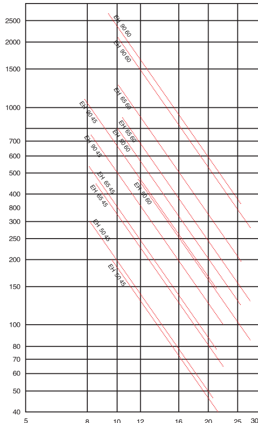
固有频率Hz
