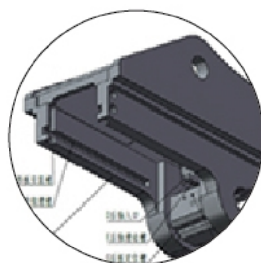
双层滑槽设计 DOUBLE LAYER SLIDING GROOVE DESIGN
