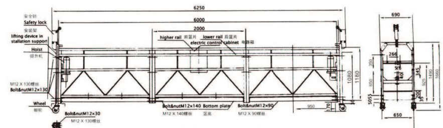
ZLP630型工作平台 ZLP630 type working platform
