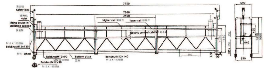
ZLP800型工作平台 ZLP800 type working platform
