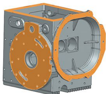
Output box
