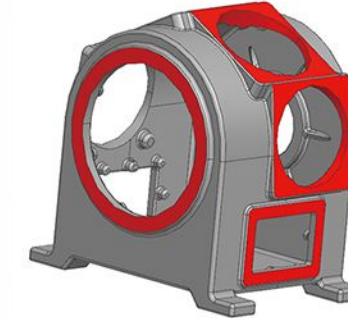
泵体
