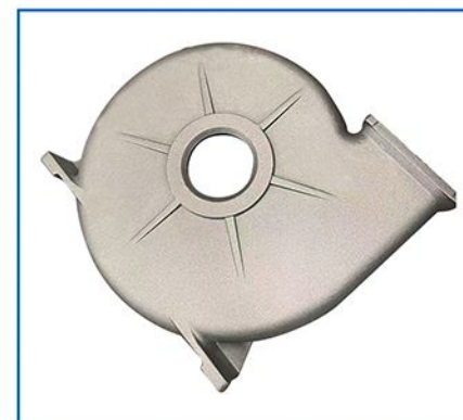
风机外壳
