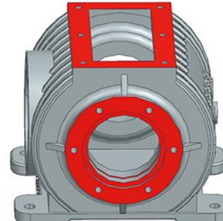
8模箱体
