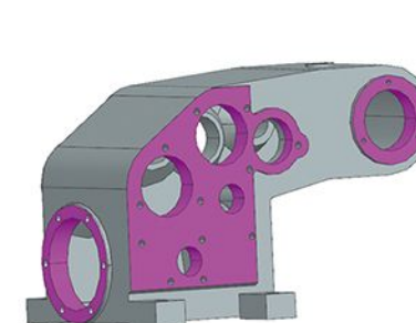
加长摘穗箱
