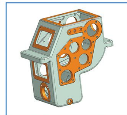
箱体
