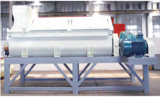
▲ 加长型搅拌主机设计，保证足够长的搅拌时间，沸腾式搅拌，大大提高搅拌匀质性
