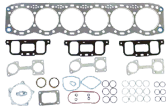
S60发动机上修理包(简配)23536442 Upper Gasket Kit
