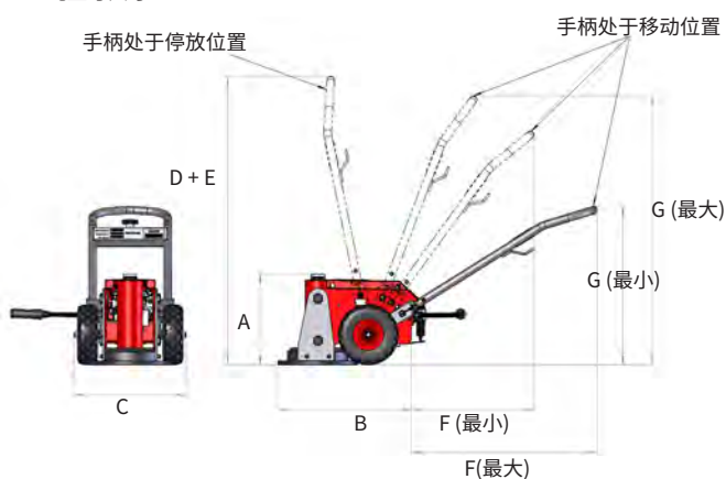
所有其他型号的尺寸:
