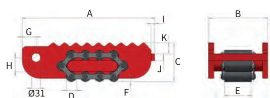
RSN60 和 RSN80的展示图
