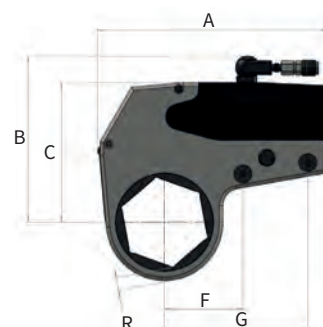
TWH430N(钢制机体)
