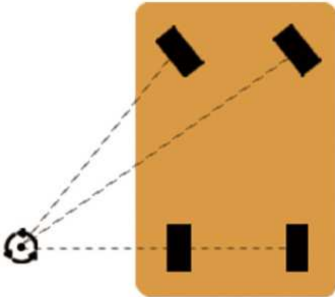
左转 Turn left
