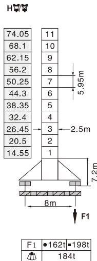
行走式 Traveling
