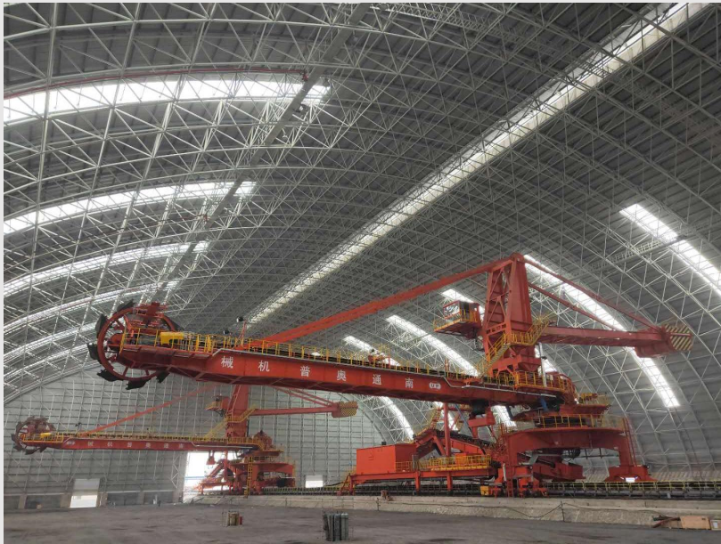
传统型斗轮堆取料机 (固定尾车、折返尾车、双尾车) 电力、钢铁、焦化应用
