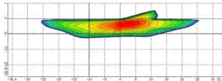
近光光型
