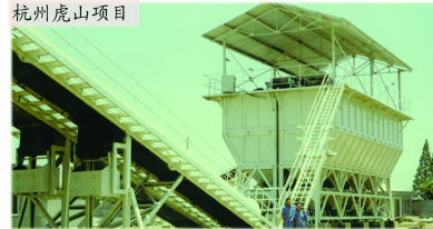
带防雨棚特殊设计
