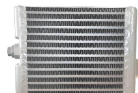
Oil Cooler 04230095 Deutz 913-914
