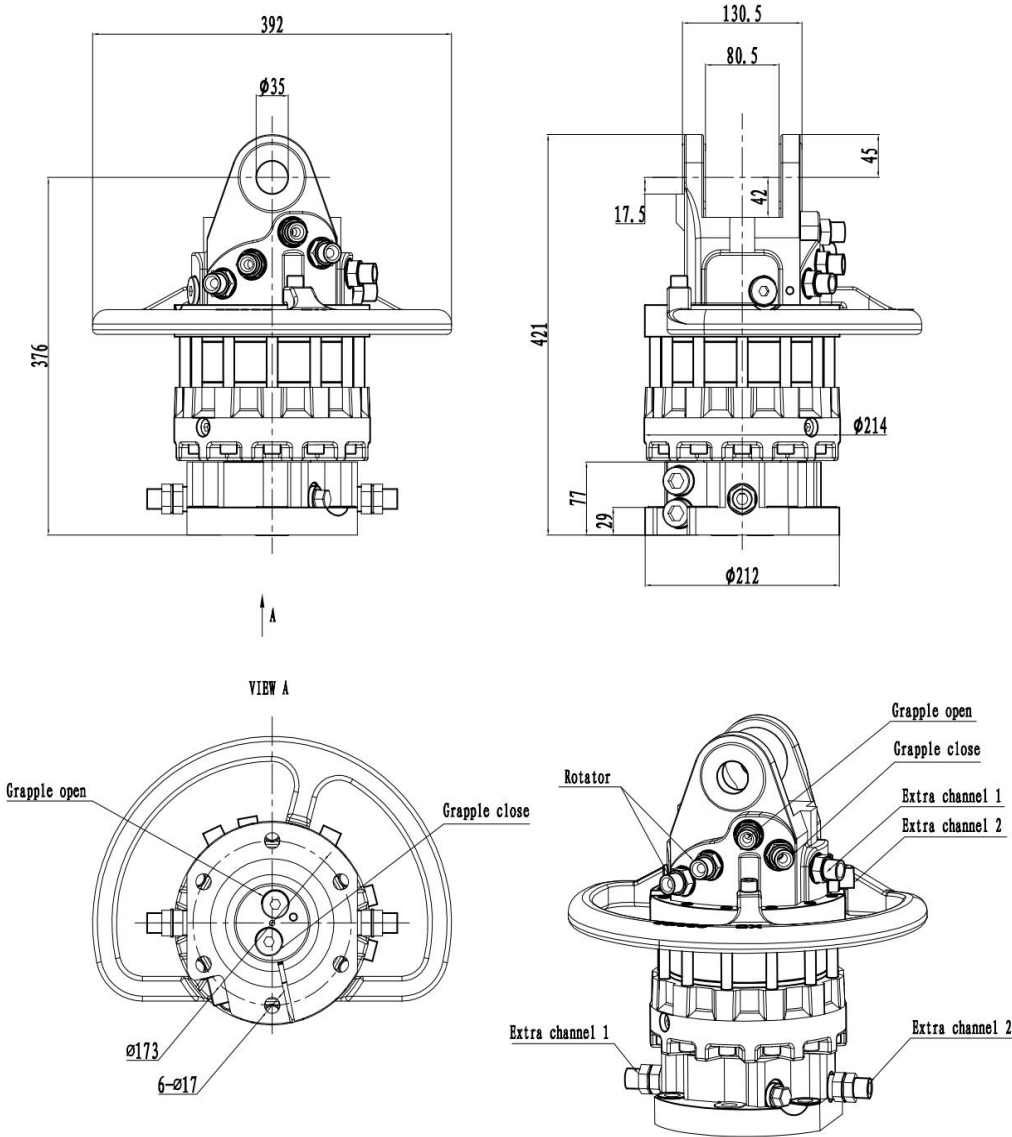
外形图 Outline Drawing
