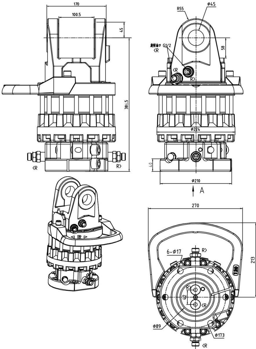
外形图 Outline Drawing
