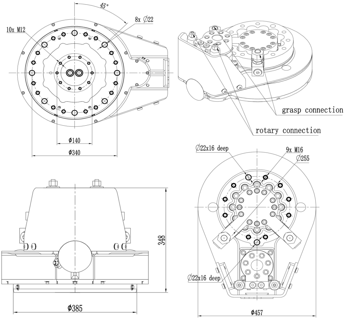
外形图 Outline Drawing
