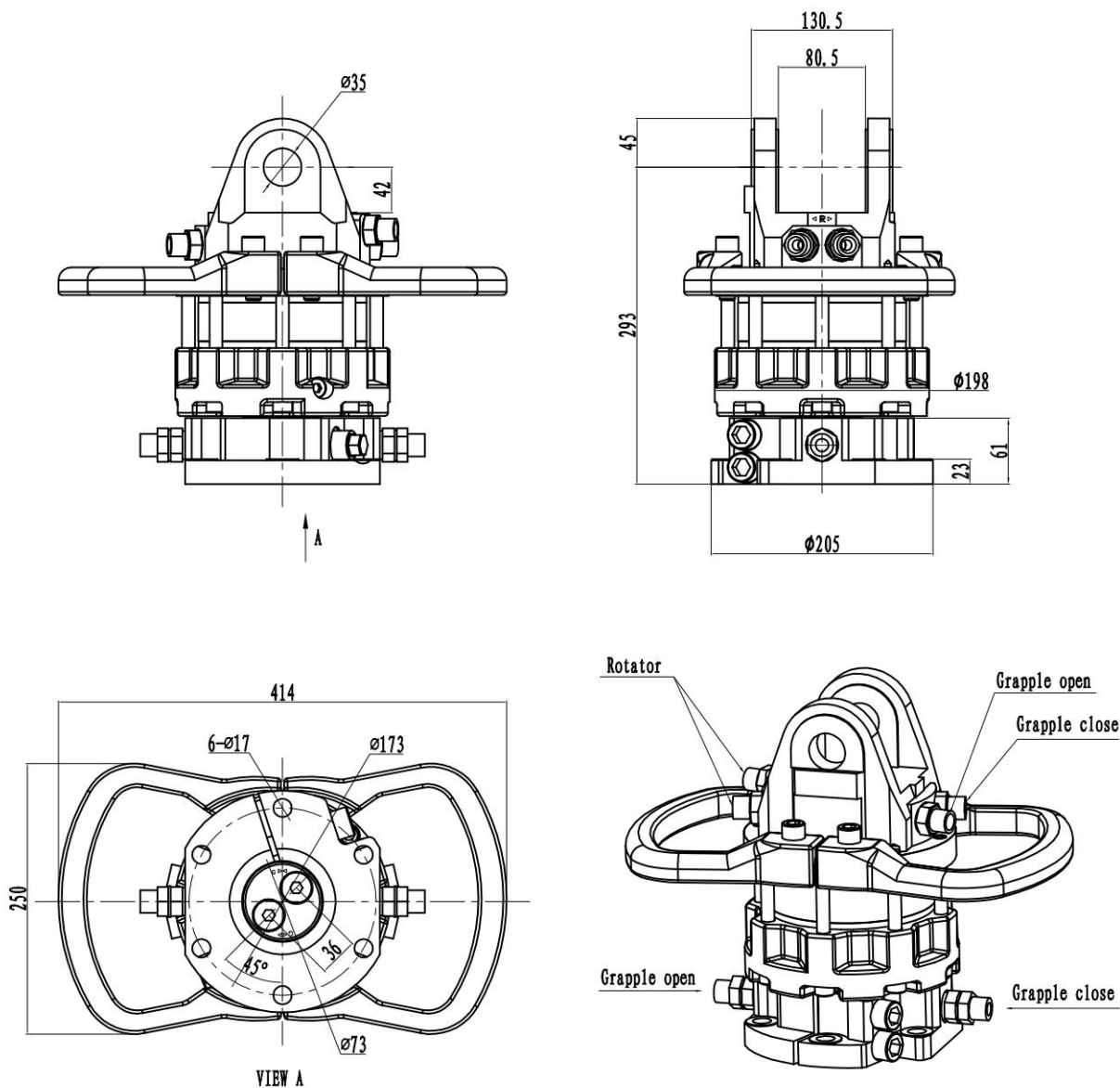
外形图 Outline Drawing
