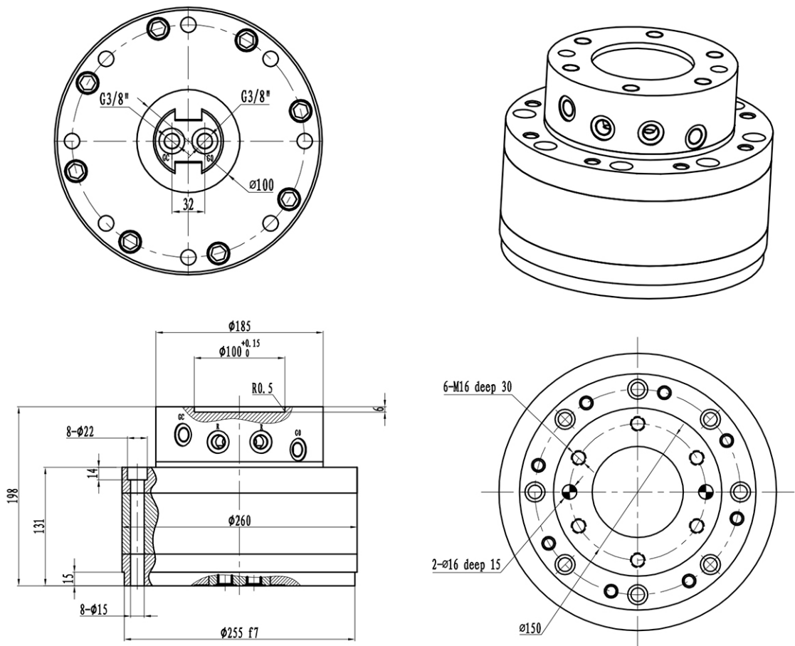
外形图 Outline Drawing
