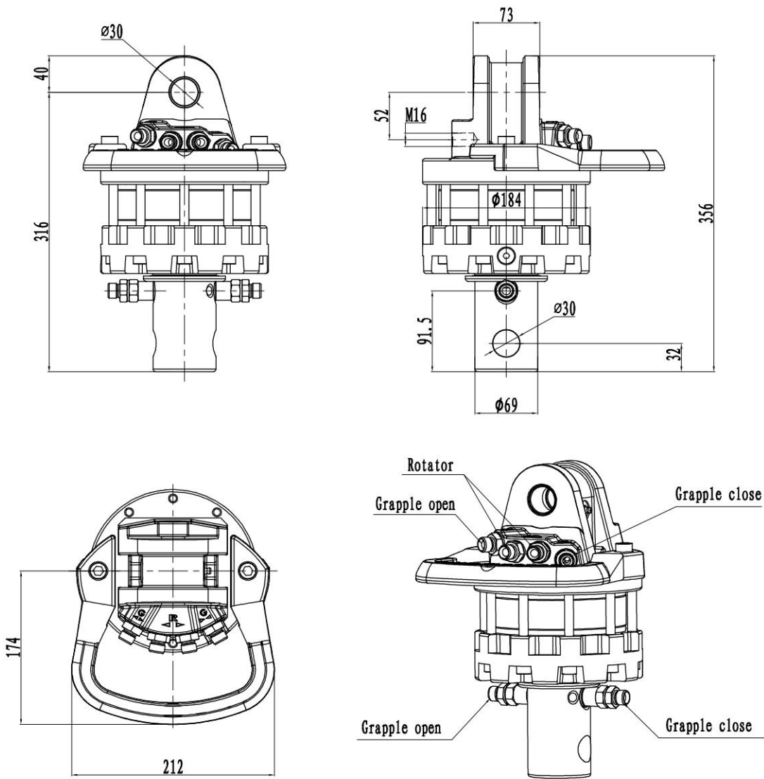
外形图 Outline Drawing
