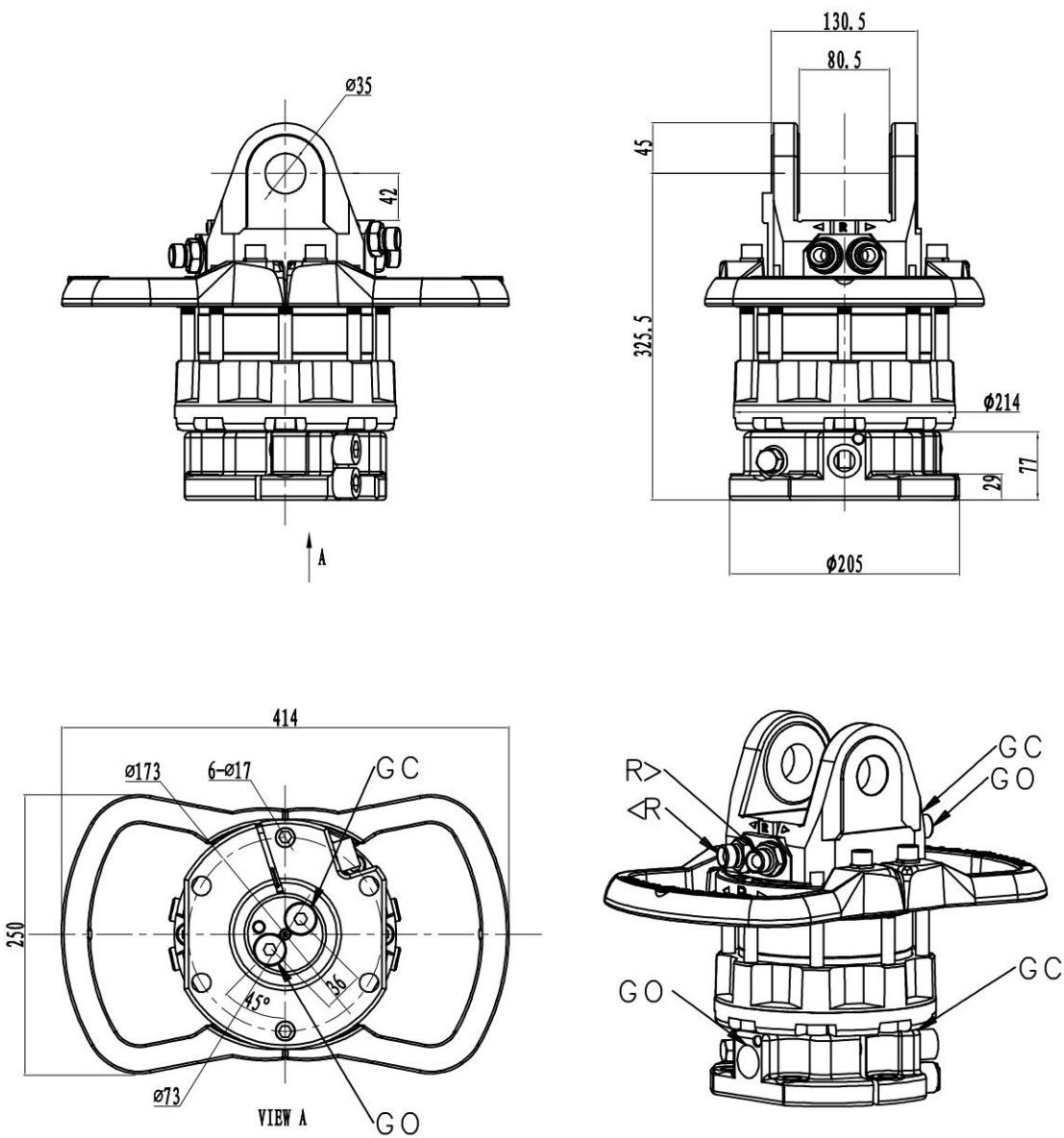
外形图 Outline Drawing
