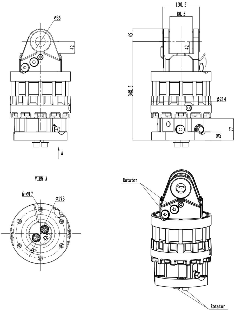
外形图 Outline Drawing
