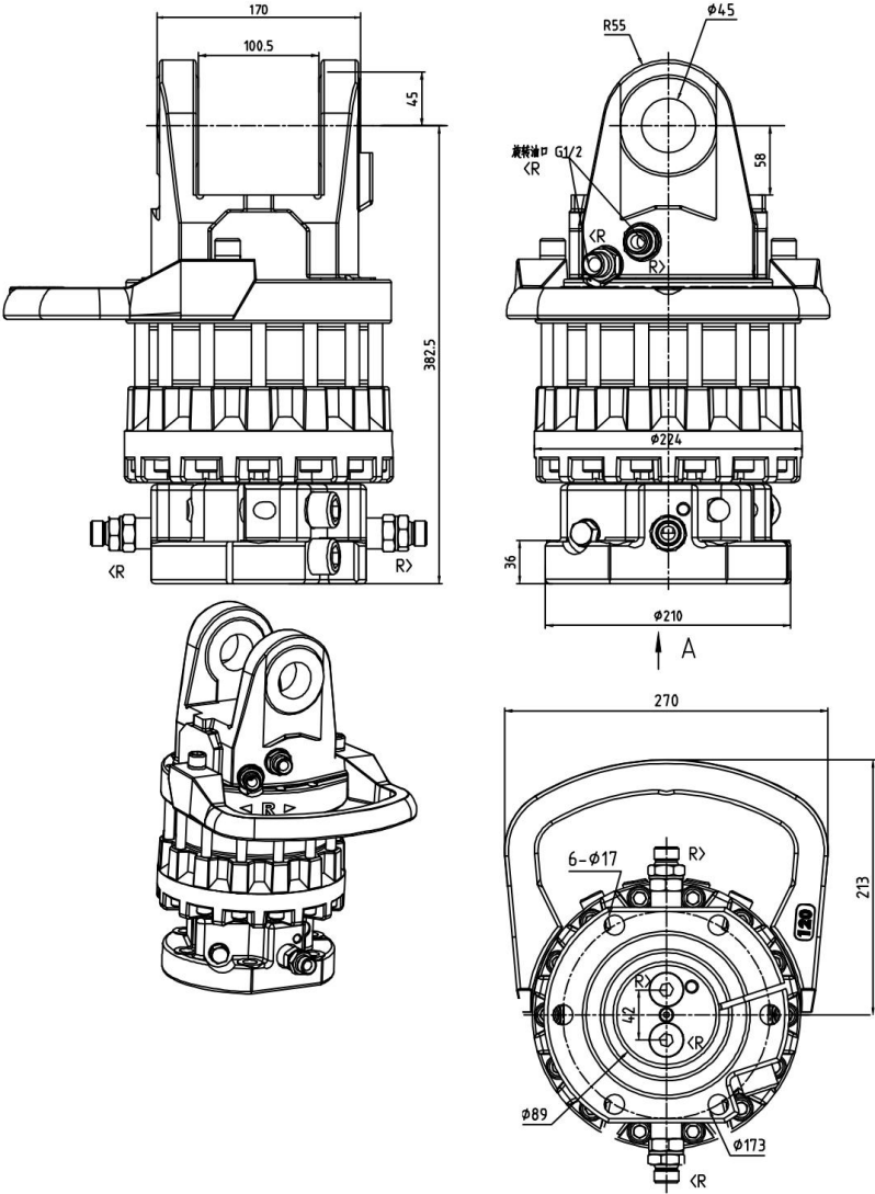
外形图 Outline Drawing
