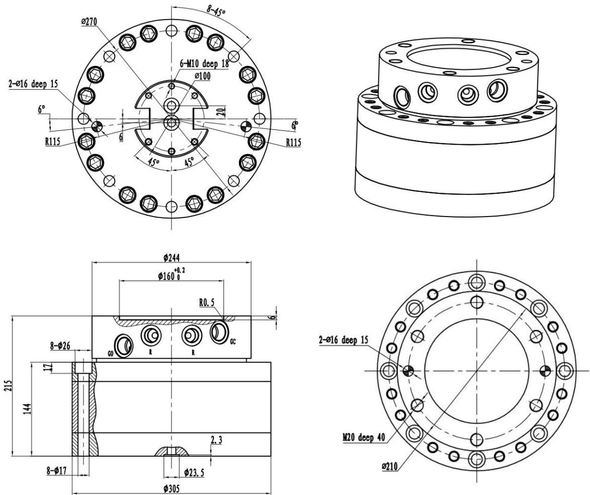
外形图 Outline Drawing
