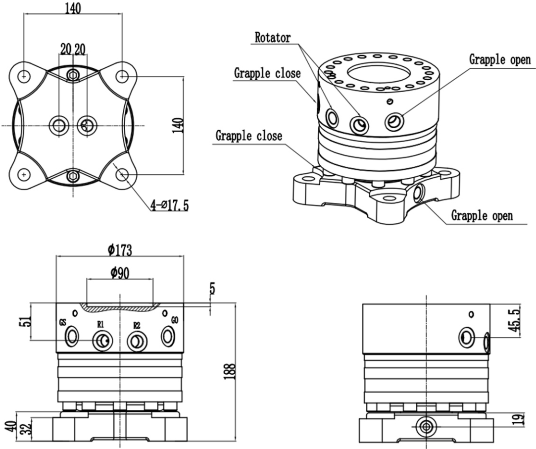
外形图 Outline Drawing
