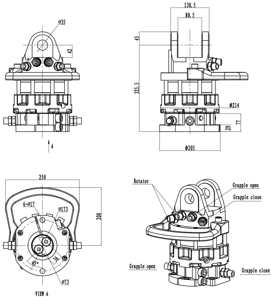
外形图 Outline Drawing
