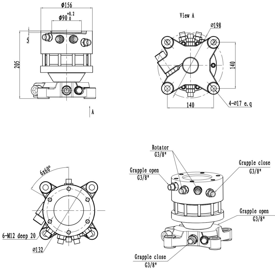
外形图 Outline Drawing
