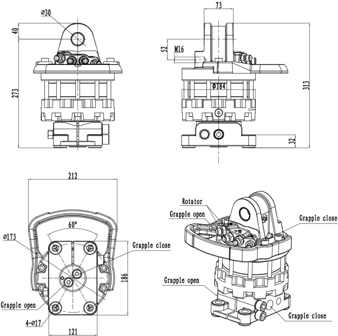
外形图 Outline Drawing
