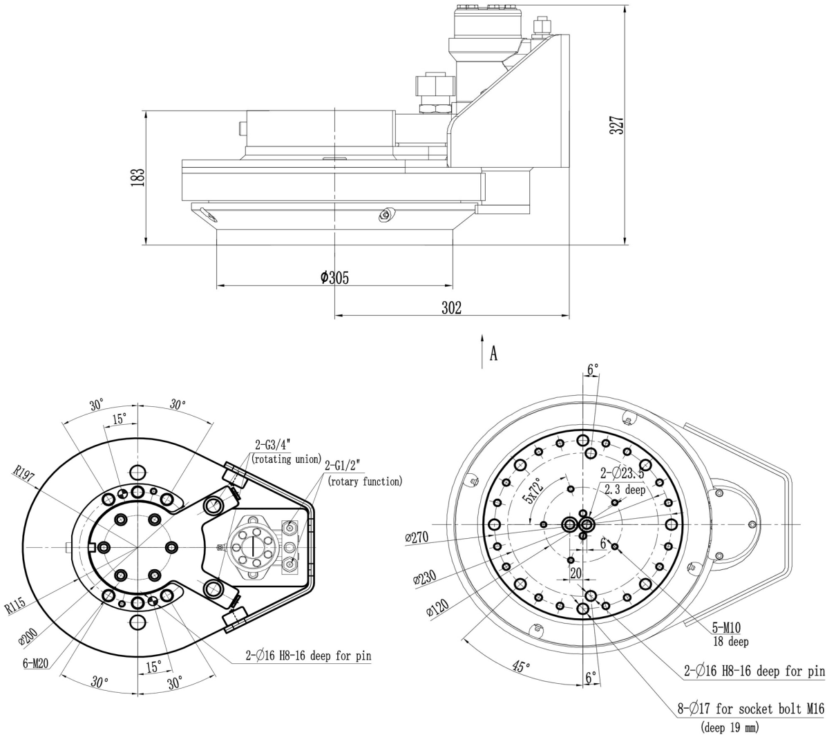
外形图 Outline Drawing
