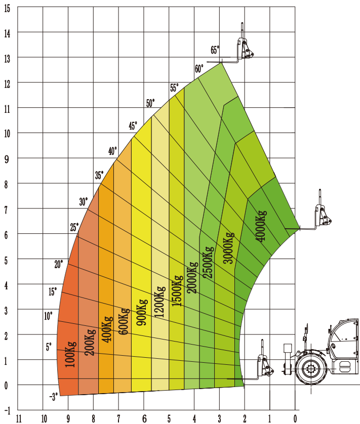
T4014载荷表(支腿收起)
