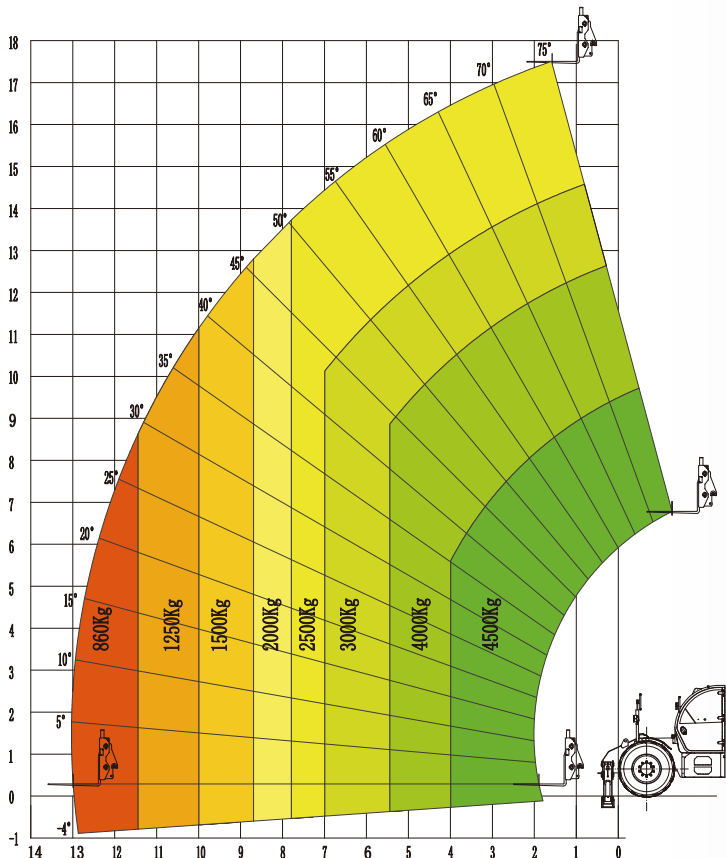
T4517载荷表(支腿放下)
