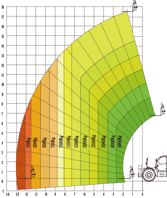
T5018载荷表(支腿收起)
