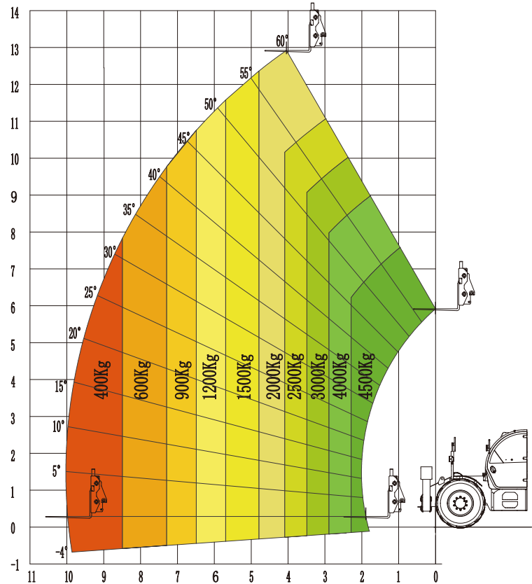
T4517载荷表(支腿收起)
