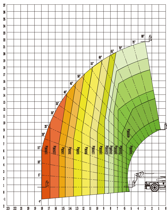
RT6025载荷表(支腿收起)
