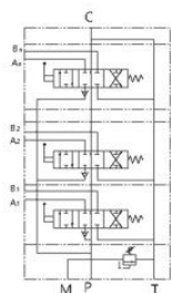
手控 Manual control
