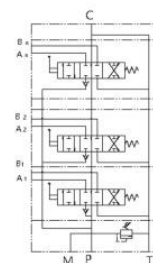
手控 Manual control
