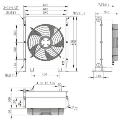
产品参数 PRODUCT PARAMETERS
