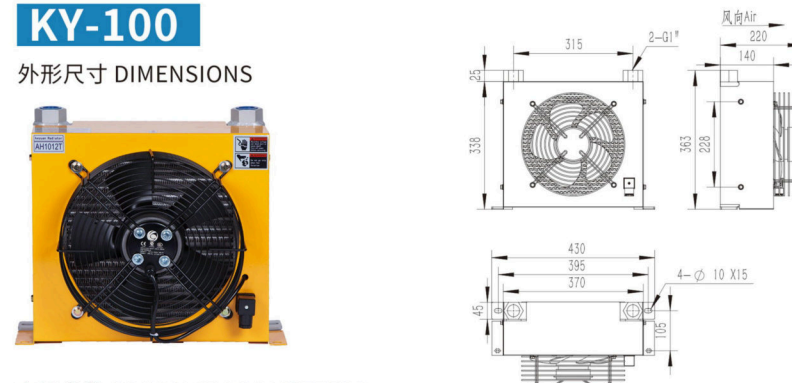
产品参数 PRODUCT PARAMETERS
