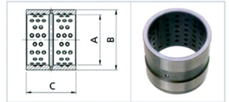
Groove Type. 6
