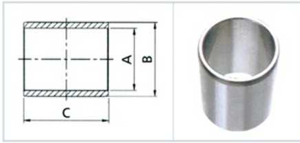
Groove Type. 1
