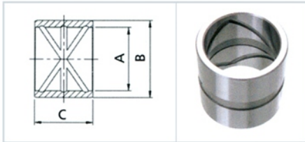
Groove Type. 4
