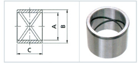
Groove Type. 3
