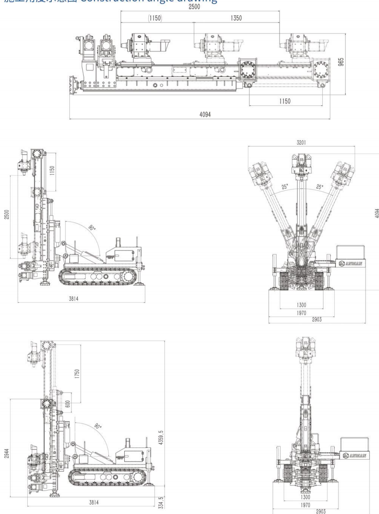
施工角度示意图 Construction angle drawing
