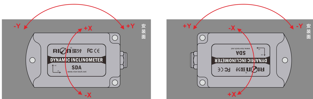
垂直向左安装
