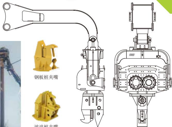
波浪桩夹嘴
