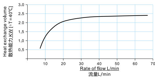
Heat diffusion function 散热性能
