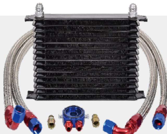
发动机油冷 261- 零件
