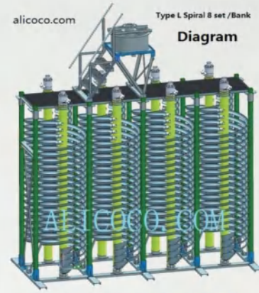
L型螺旋溜槽机组框架示意图
