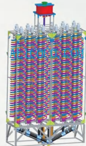
FG7型螺旋选矿机组框架示意图
