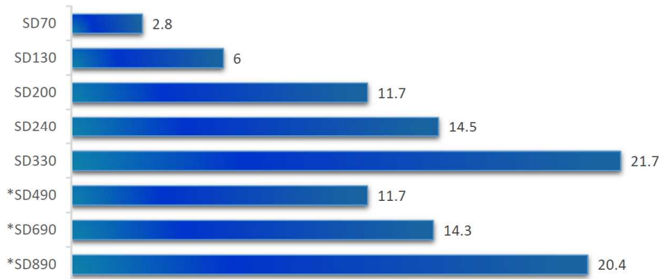
输出扭/kNm
