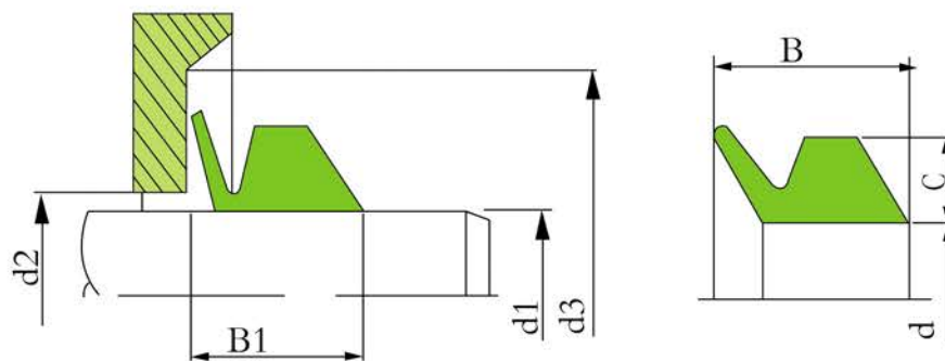
尺寸表
