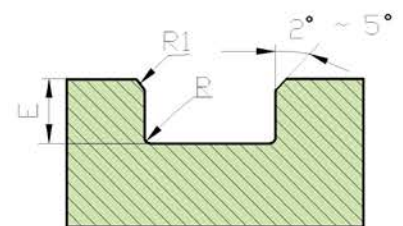
b矩形沟槽 (1)
