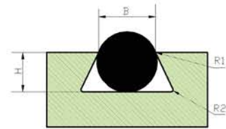
C梯形沟槽
