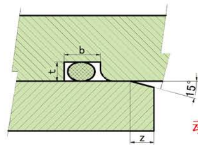
O型圈/星型圈以液體作為介質時開槽尺寸建議參數 (動態)
