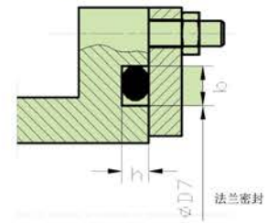
b矩形沟槽 (4)
