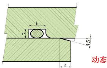
O型圈/星型圈以氣體作為介質時開槽尺寸建議參數（動態2）
