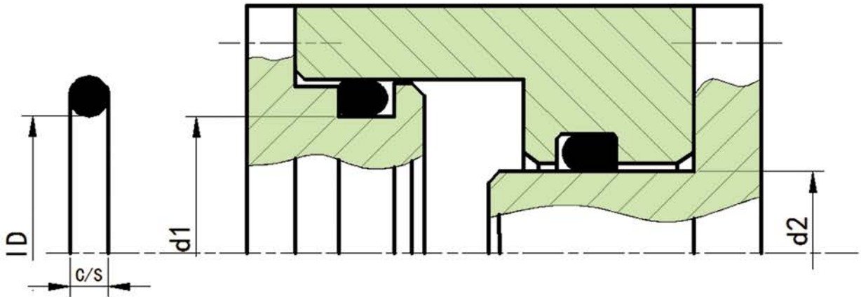
徑向安裝，靜密封和動密封
