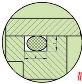
O型圈/星型圈開槽尺寸建議參數 (靜態)
