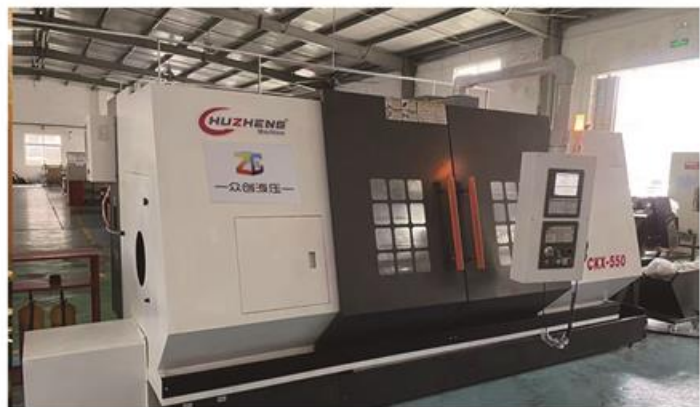
▼ 超长深孔液压缸筒珩磨辊压机
