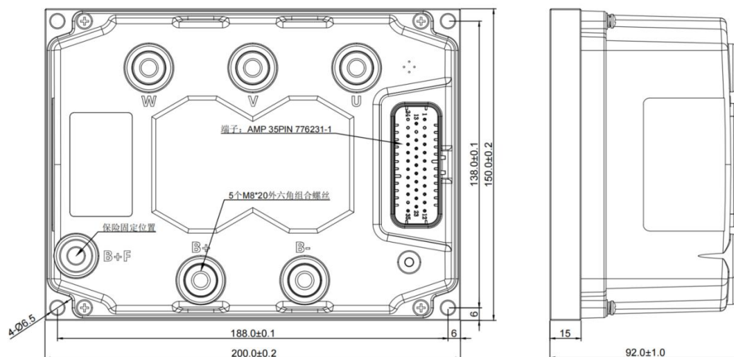
图 2.1.1 安装尺寸
