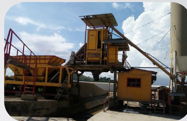
YHZS50 in Papua New Guinea
