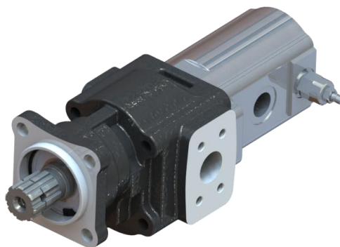
GP40/SP20 双联泵
