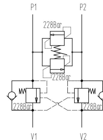
平衡阀+双向溢流阀 可选平衡阀液压原理图
