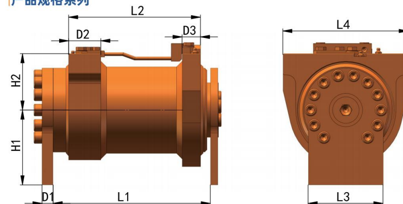
BQ8系列挖掘机摆动油缸选型
