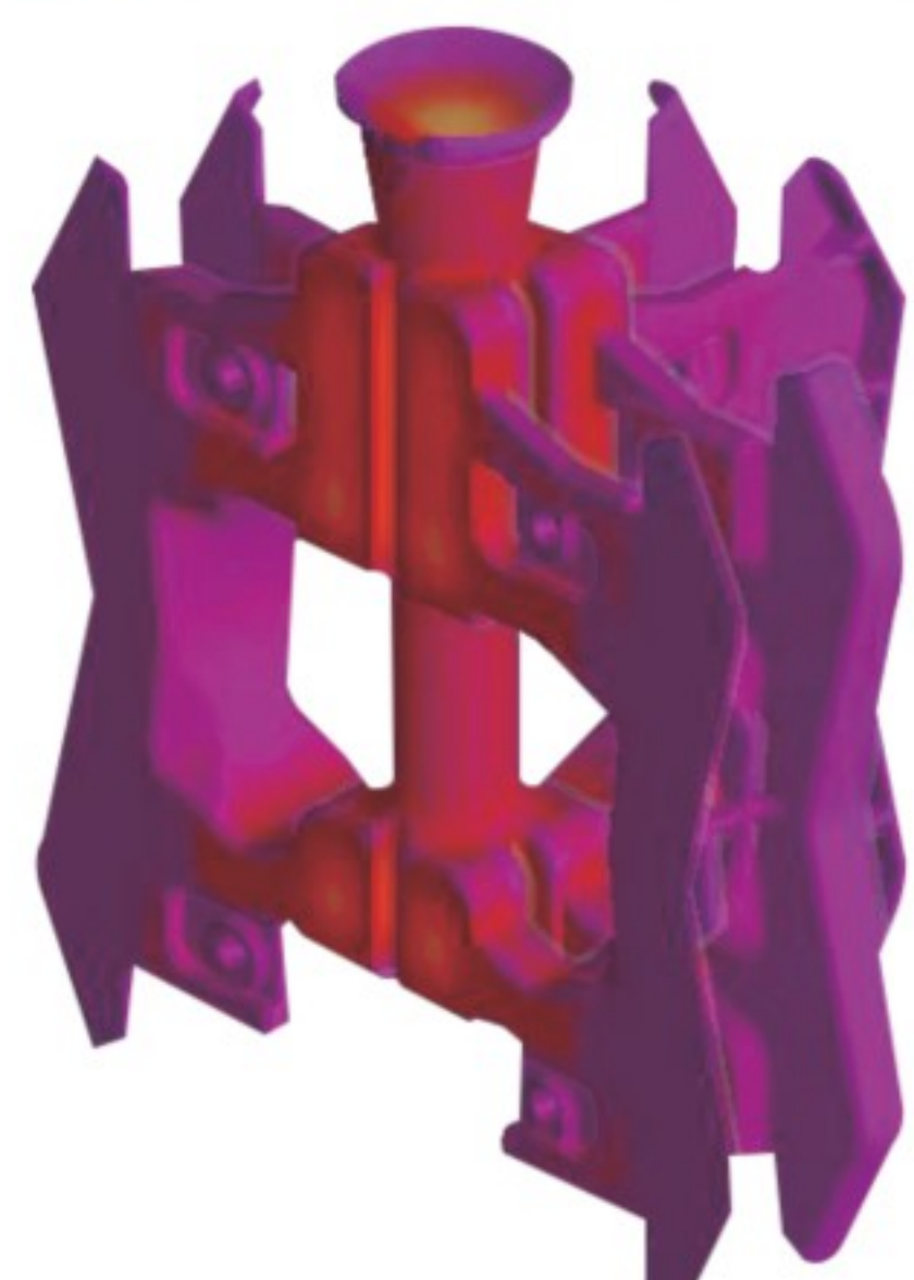
模拟铸造 NOVACAST
