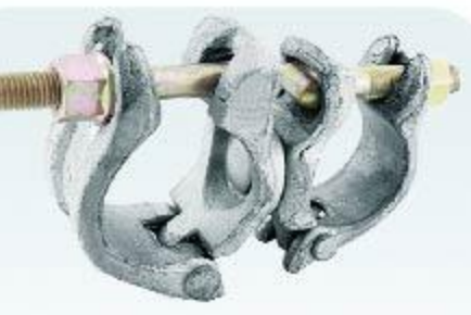
RFH-A053 旋转扣件 Swivel Coupler 60X48.3mm 1.60kg
