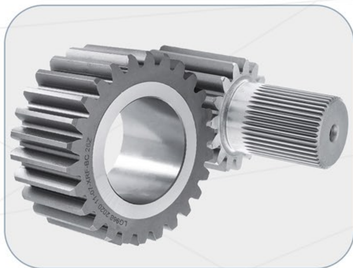
临工968, 26齿 行星轮 太阳轮
