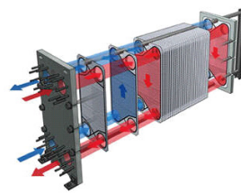
板式水冷散热器
