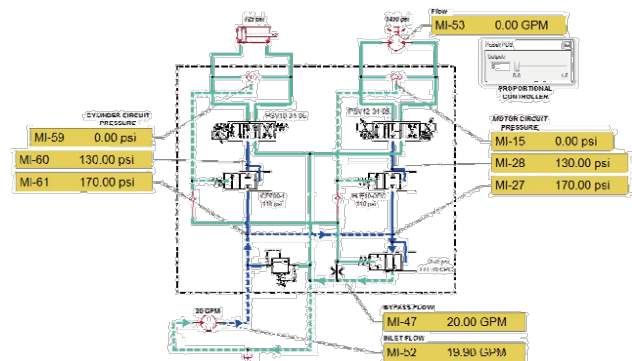
液压系统仿真
