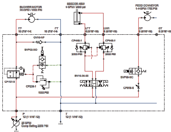
液压系统原理
