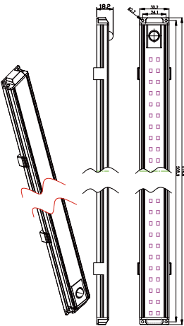
红外感应开关 PIR SENSOR
