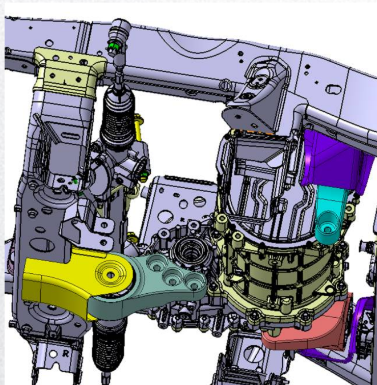
电机悬置总布置
