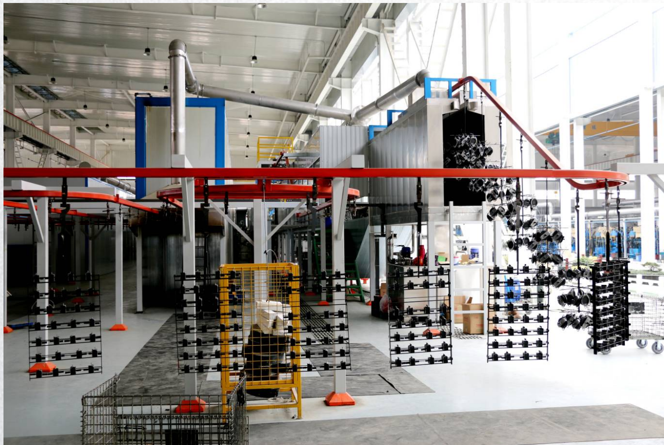
电泳涂装流水线
