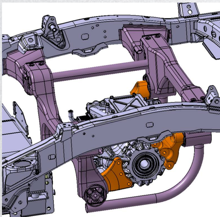
电机悬置总布置
