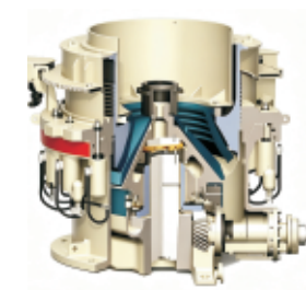
SM Series Cone Crusher SM 系列圆锥破碎机
