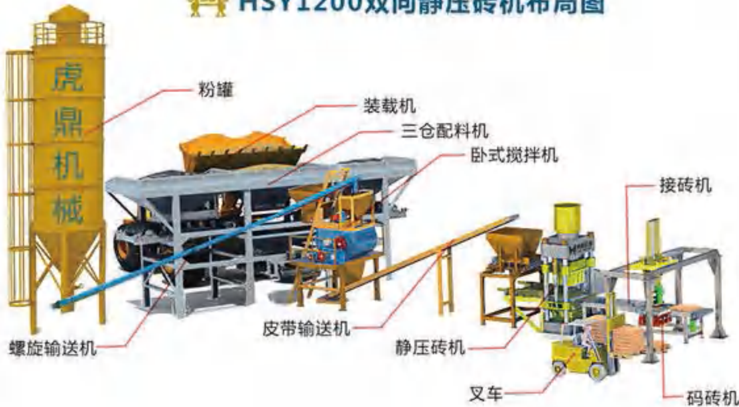
虎鼎机械 HSY1200双向静压砖机布局图
