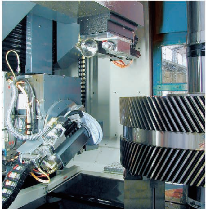
人字齿齿轮 Herringbone Gear
