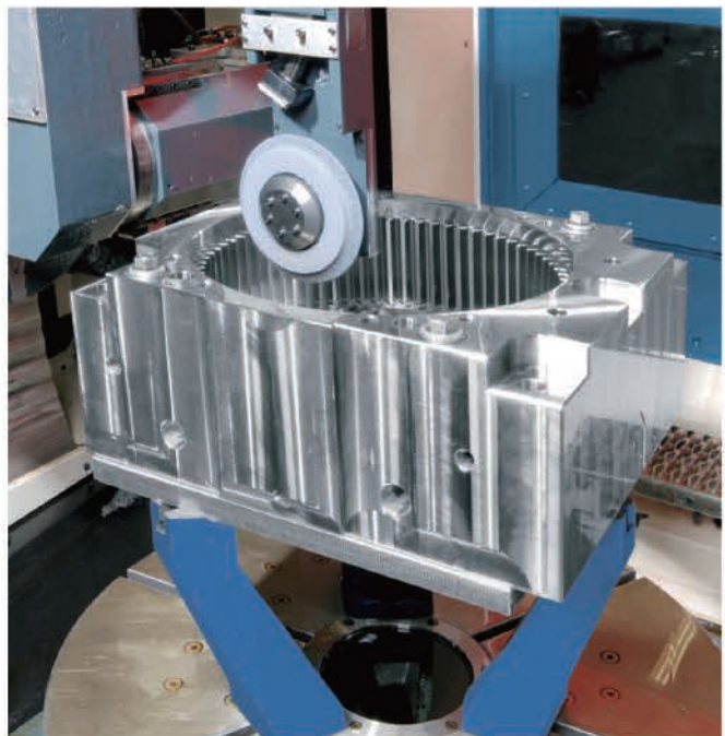
内轮 Inner Gear
