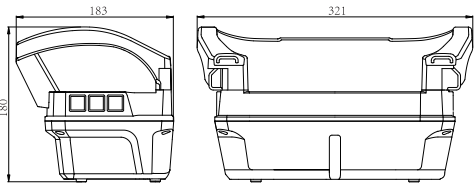
FYF20C、FYF100A尺寸图
