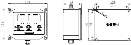
FYS20C尺寸图
