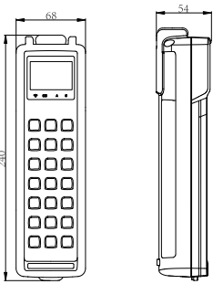
FYF20B尺寸图
