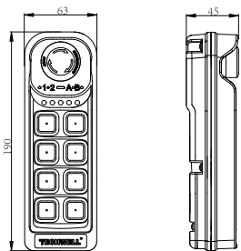
BEA尺寸图
