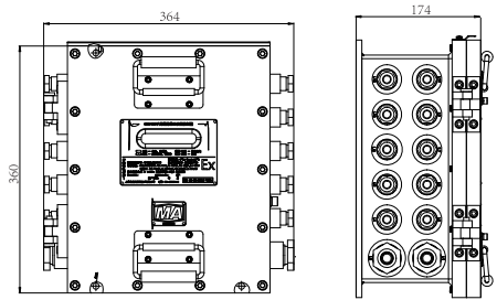
KXJ127尺寸图
