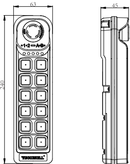
BTA尺寸图
