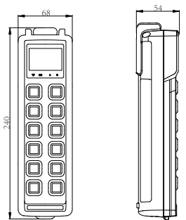
BTB尺寸图
