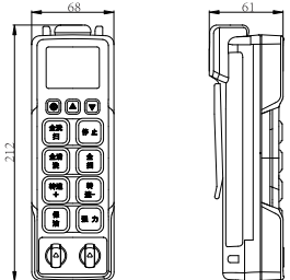
BEB尺寸图
