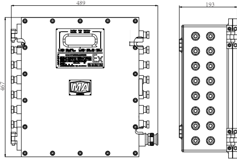
KXJ1140尺寸图
