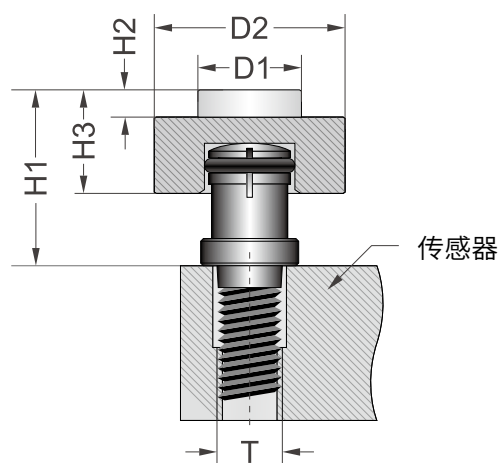
尺寸 | Dimensions
