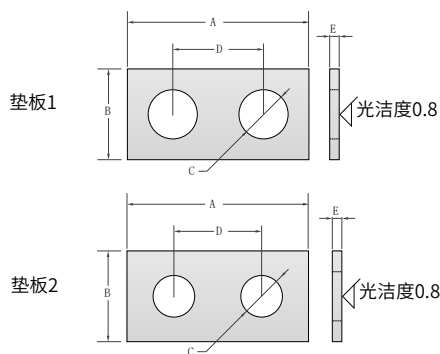
尺寸 | Dimensions
