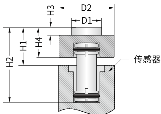
尺寸 Dimensions
