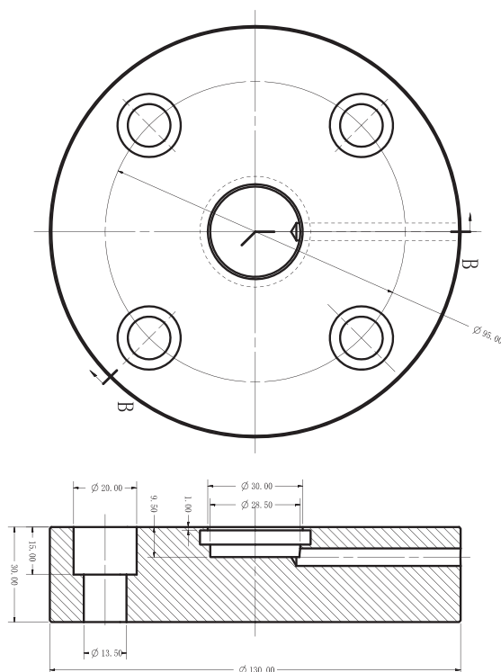
尺寸 | Dimensions
