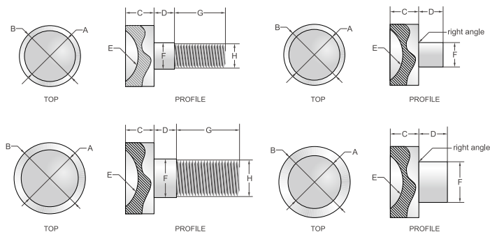
尺寸 | Dimensions
