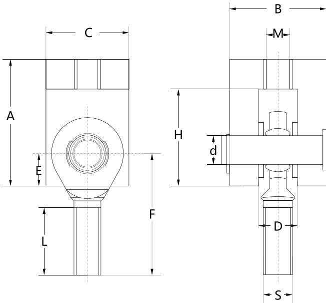
尺寸 | Dimensions
