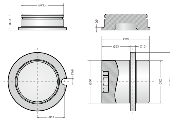
尺寸 | Dimensions
