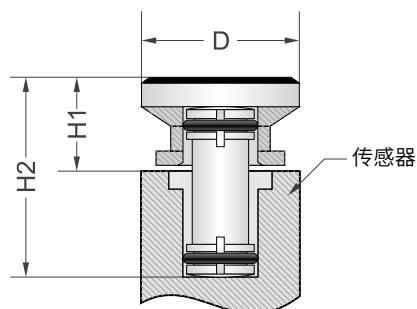
尺寸 Dimensions
