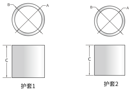
尺寸 | Dimensions
