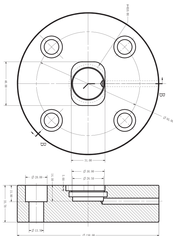
尺寸 | Dimensions
