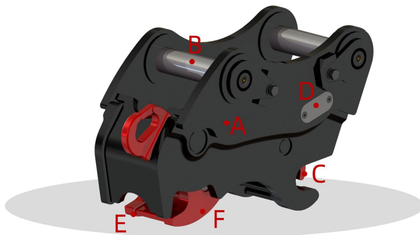
E: 后保险锁 活动钩带主弹簧保险锁， 以防油缸内泄，活动钩 回缩。
