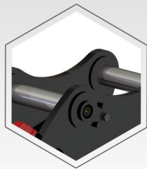
B: 上部轴 42CrMo热处理销轴， 24-28HRC，高频 50-55HRC，硬度高， 更耐磨。
