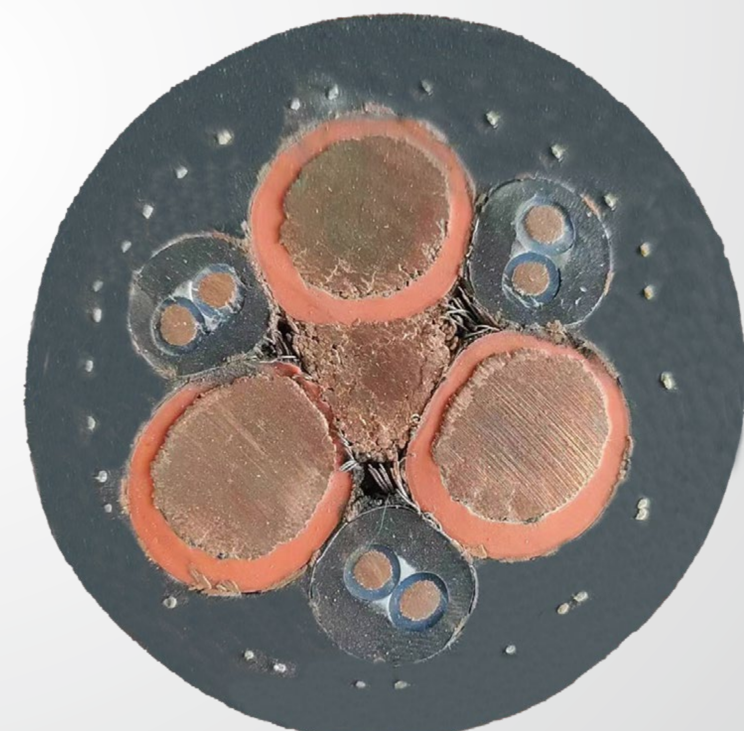
MCPT 1.9 / 3.3KV 双层护套凯夫拉编织加强型
