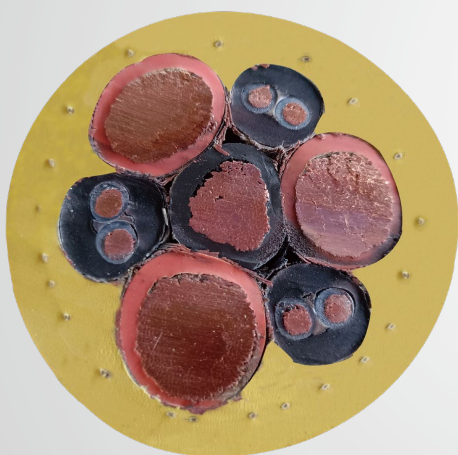
MCPT 0.66 / 1.14KV 双层护套凯夫拉编织加强型
