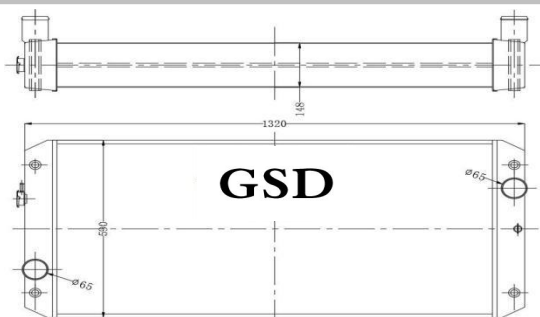
挖机全铝水箱 外形: 1320×595×170 水口: \phi 65
