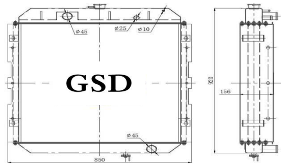
挖机全铝水箱 外形: 920×850×156 水口: \phi 45
