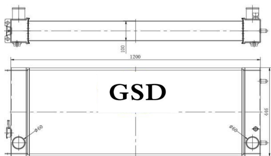
挖机全铝水箱 外形: 1210×450×126 水口: Φ60
