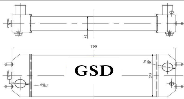
挖机全铝水箱 外形: 790×260×110 水口: \phi 50
