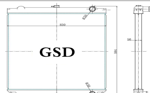
挖机全铝水箱 外形: 980×830×85 水口: \phi 50
