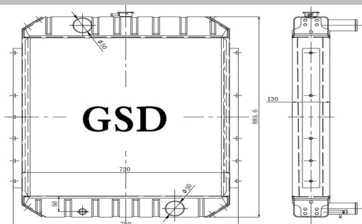
挖机全铝水箱 外形: 890×720×130 水口: \phi 50
