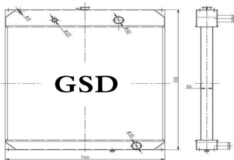
挖机全铝水箱 外形: 930×760×105 水口: \phi 45
