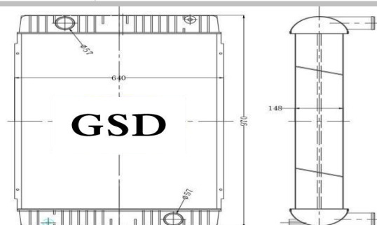
挖机全铝水箱 外形: 970×640×180 水口: \phi 58
