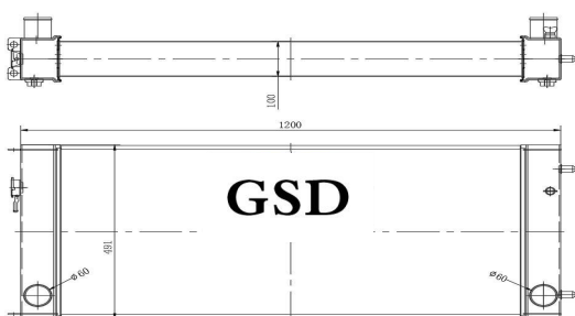
挖机全铝水箱 外形: 1200×490×126 水口: Φ60
