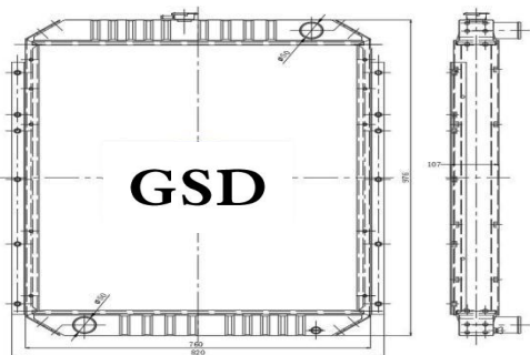
挖机全铝水箱 外形: 980×760×100 水口: \phi 50
