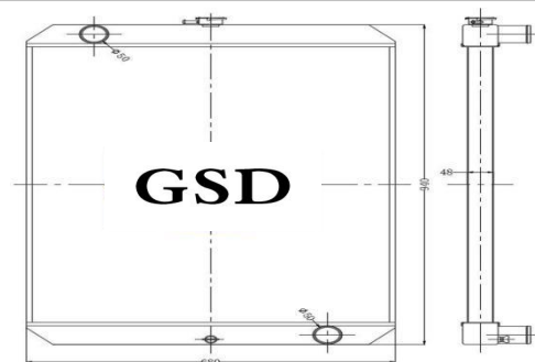
挖机全铝水箱 外形: 940×680×90 水口: \phi 50
