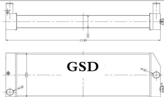
挖机全铝水箱 外形: 1140×370×140 水口: \phi 50
