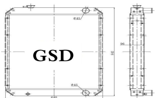
挖机全铝水箱 外形: 840×640×100 水口: \phi 45
