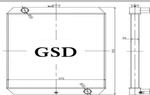
挖机全铝水箱 外形: 900×680×80 水口: \phi 50
