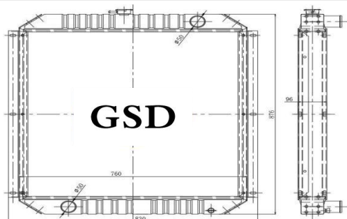
挖机全铝水箱 外形: 880×760×96 水口: \phi 50
