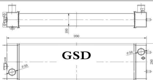
挖机全铝水箱 外形: 990×290×126 水口: \phi 50
