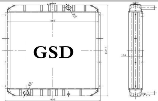
挖机全铝水箱 外形: 1150×865×135 水口: \phi 50
