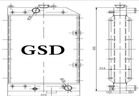
挖机全铝水箱 外形: 695×370×115 水口: \phi 38
