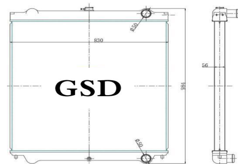
挖机全铝水箱 外形: 980×830×85 水口: Φ50
