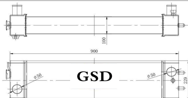
挖机全铝水箱 外形: 900×230×126 水口: \phi 50
