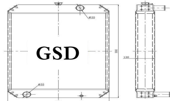
挖机全铝水箱 外形: 990×705×130 水口: \phi 55
