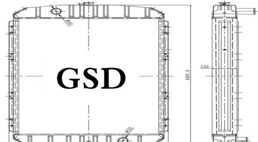
挖机全铝水箱 外形: 1190×790×135 水口: \phi 50
