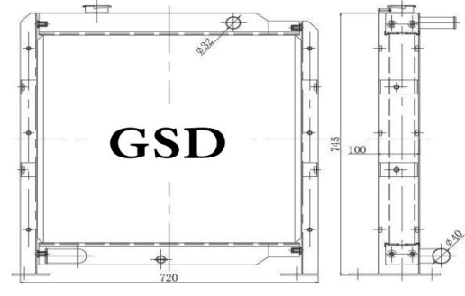
挖机全铝水箱 外形: 745×720×100 水口: \phi 32/\phi 40
