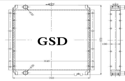
挖机全铝水箱 外形: 970×760×100 水口: \phi 50
