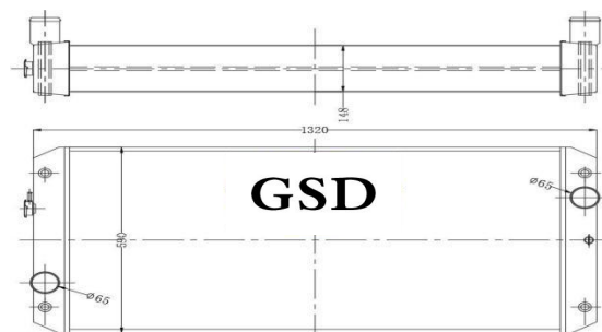
挖机全铝水箱 外形: 1320×595×170 水口: \phi 65
