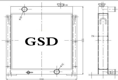
挖机全铝水箱 外形: 650×480×75 水口: Φ42
