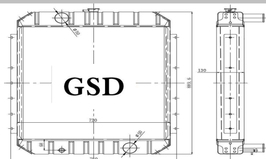
挖机全铝水箱 外形: 890×720×130 水口: \phi 50
