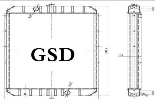
挖机全铝水箱 外形: 1150×855×135 水口: \phi 50
