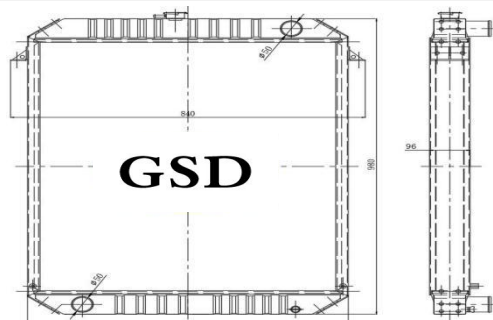
挖机全铝水箱 外形: 980×760×96 水口: \phi 50
