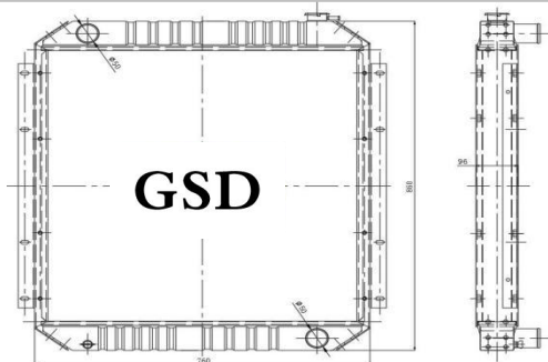
挖机全铝水箱 外形: 860×760×96 水口: \phi 50
