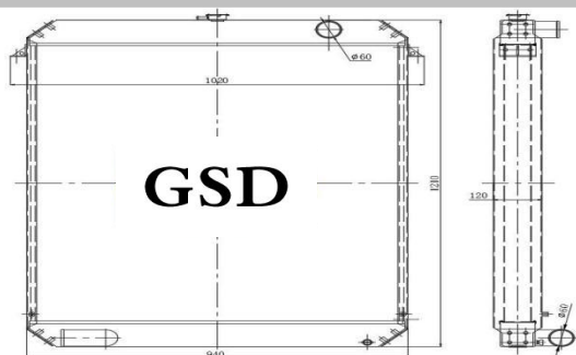
挖机全铝水箱 外形: 1210×960×120 水口: \phi 50
