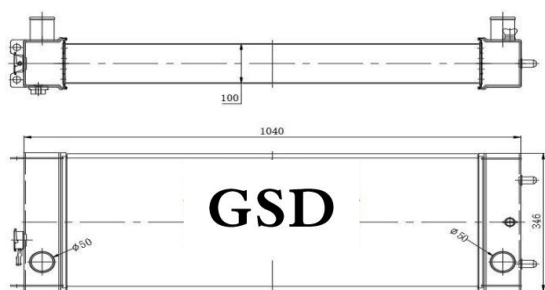
挖机全铝水箱 外形: 1040×345×125 水口: \phi 50
