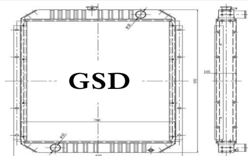
挖机全铝水箱 外形: 980×760×100 水口: \phi 50
