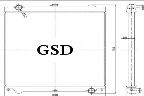
挖机全铝水箱 外形: 980×830×85 水口: \phi 50
