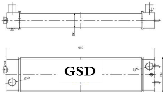
挖机全铝水箱 外形: 970×250×126 水口: \phi 50
