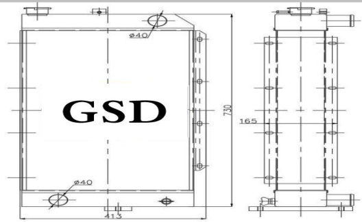
挖机全铝水箱 外形: 730×380×120 水口: Φ40
