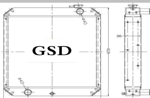
挖机全铝水箱 外形: 670×560×96 水口: \phi 40
