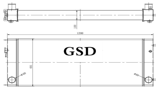
挖机全铝水箱 外形: 1200×490×126 水口: Φ60
