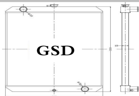
挖机全铝水箱 外形: 900×680×70 水口: \phi 50
