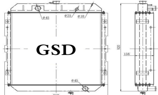
挖机全铝水箱 外形: 920×850×156 水口: \phi 45
