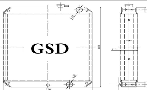
挖机全铝水箱 外形: 680×550×110 水口: \phi 38
