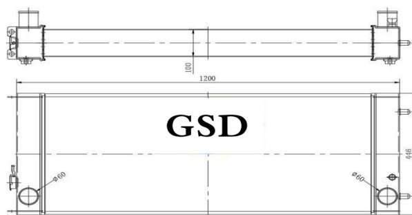
挖机全铝水箱 外形: 1200×450×126 水口: \phi 60
