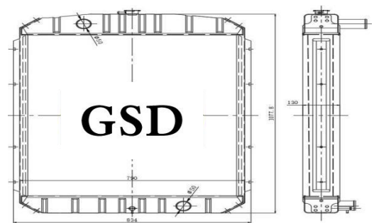
挖机全铝水箱 外形: 1080×790×130 水口: \phi 50
