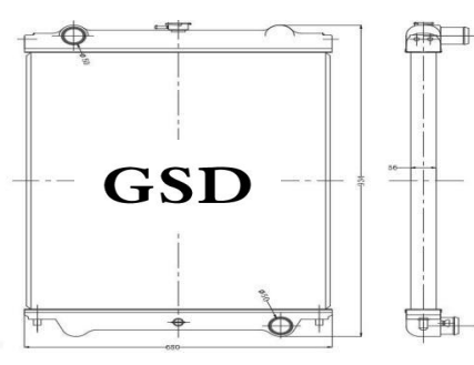
挖机全铝水箱 外形: 930×680×90 水口: Φ50
