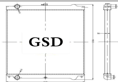
挖机全铝水箱 外形: 1075×830×90 水口: \phi 50
