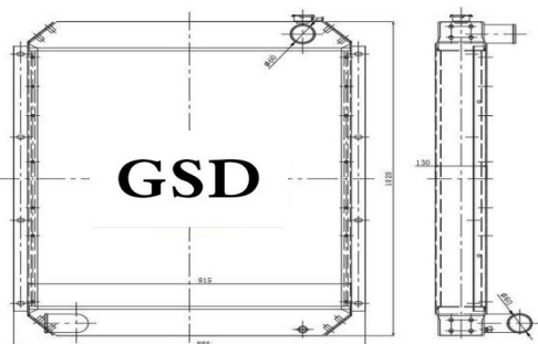
挖机全铝水箱 外形: 1020×815×130 水口: \phi 60
