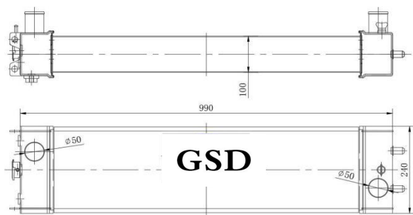
挖机全铝水箱 外形: 990×240×126 水口: \phi 50
