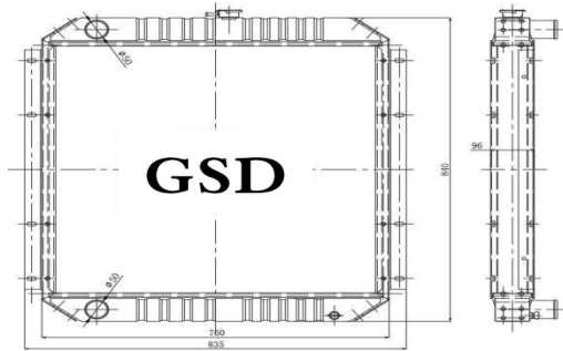
挖机全铝水箱 外形: 840×760×96 水口: φ 50
