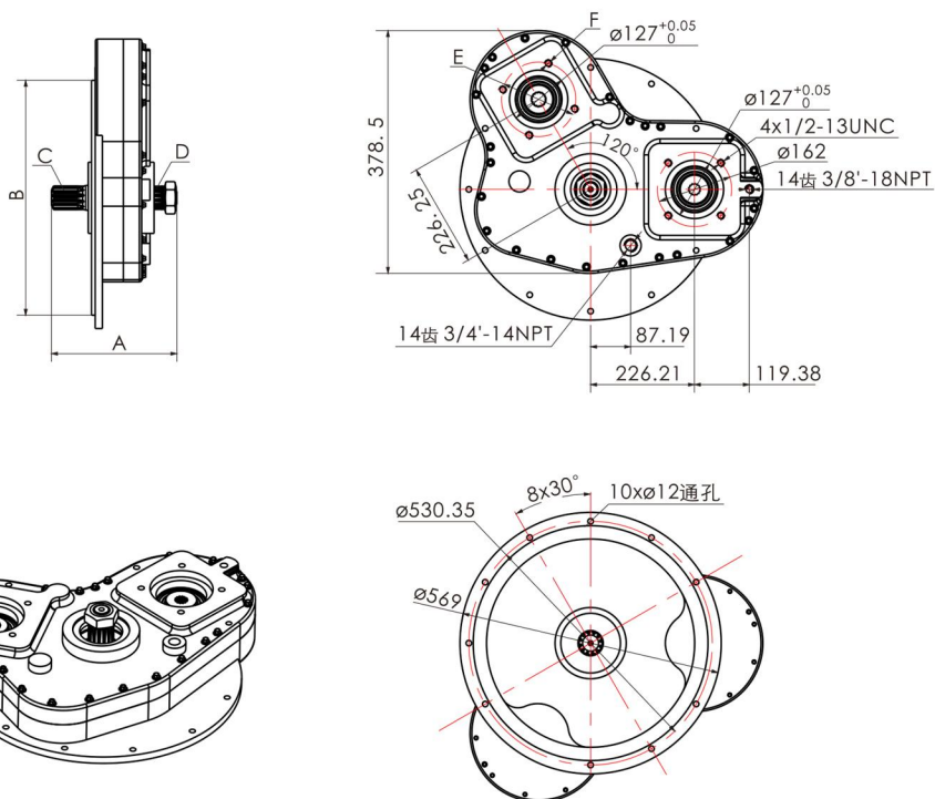
WHL系列安装尺寸图
