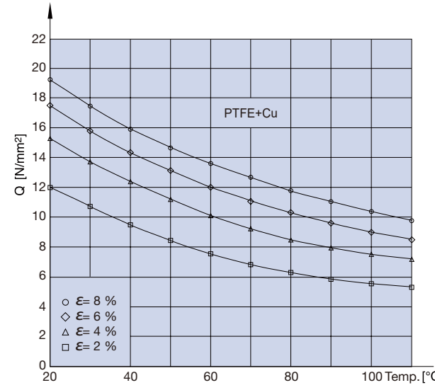
S1106材料在不同温度和压缩变形率的许可载荷
