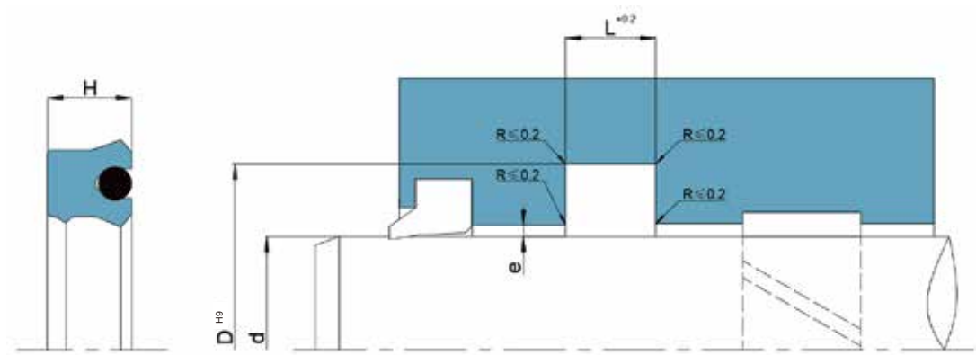
备注：间隙e请参照“密封沟槽设计”章节
