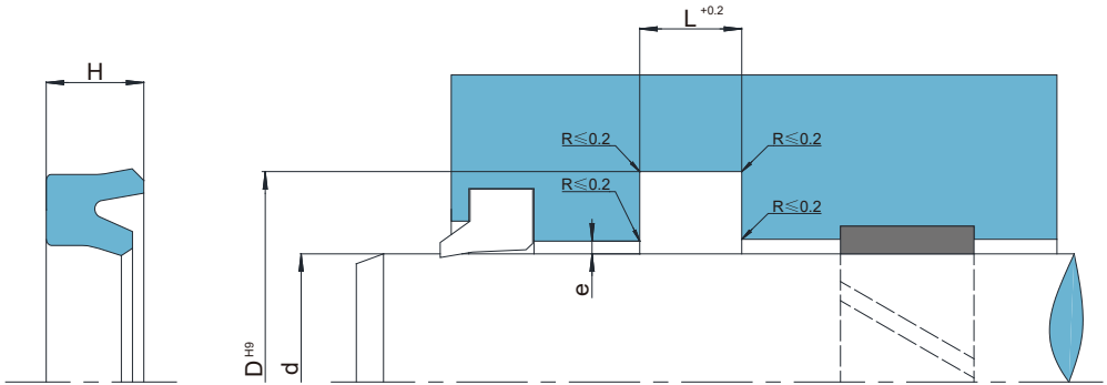
备注：间隙e请参照“密封沟槽设计”章节
