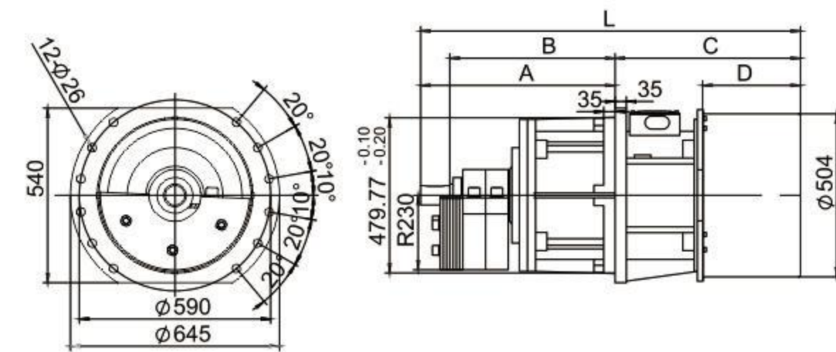
图6 侧板振动电机外形安装图 (SIZE105 A)
