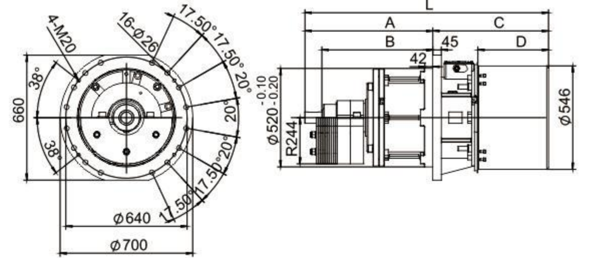
图7 侧板振动电机外形安装图 (SIZE110 B)
