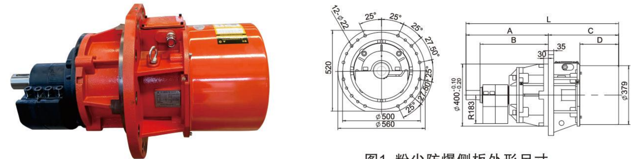
图1 粉尘防爆侧板外形尺寸
