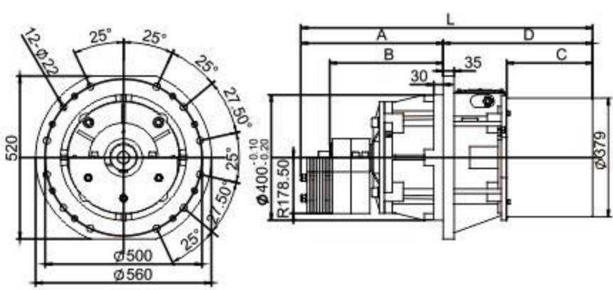
图3 侧板振动电机外形安装图 (SIZE90 91 A)
