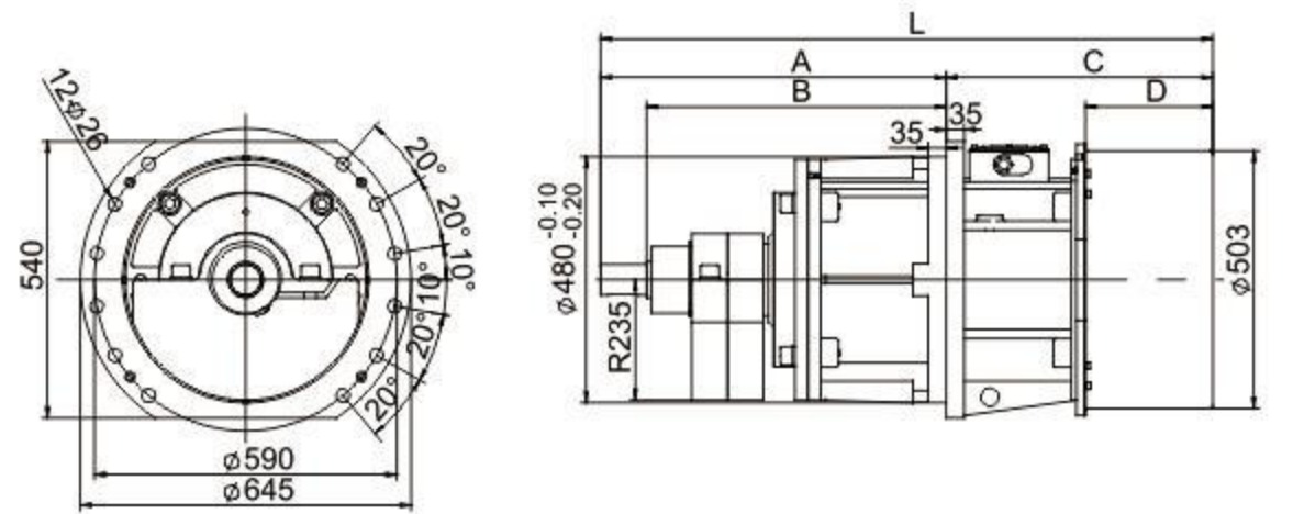
图5 侧板振动电机外形安装图 (SIZE105 B)
