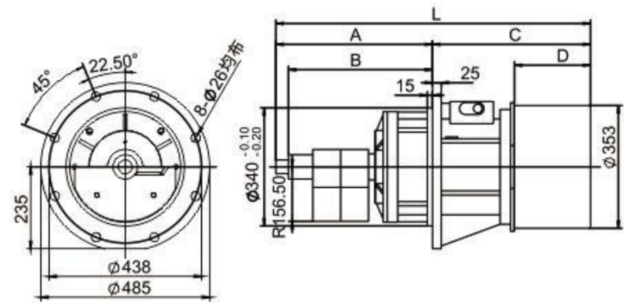
图2 侧板振动电机外形安装图 (SIZE85BE B)
