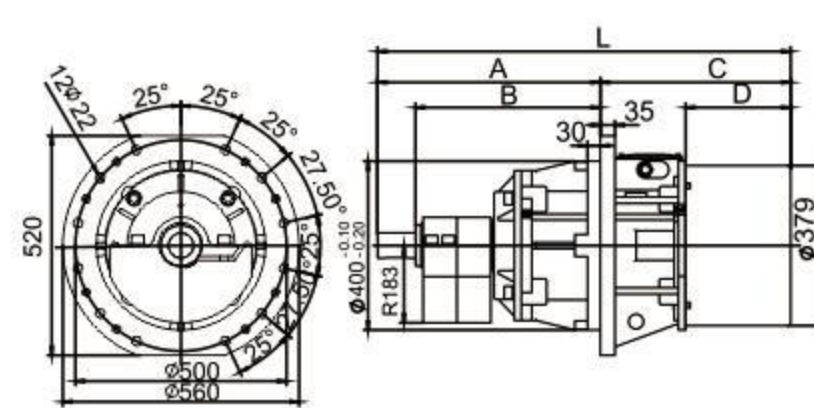
图4 侧板振动电机外形安装图 (SIZE90 91 B)
